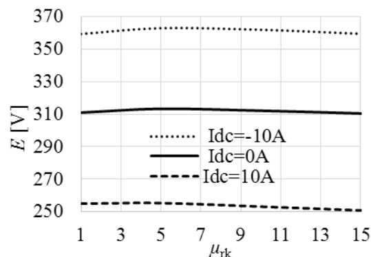
Rys. 10. Zależność wartości skutecznej SEM w zależności od przenikalności magnetycznej klinów oraz prądu zasilania dodatkowej cewki
