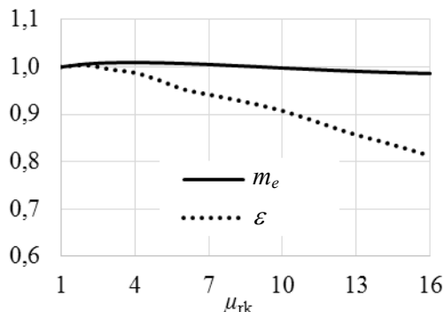
Rys. 8. Zmiana względnej wartości momentu elektromagnetycznego m_e i względnego współczynnika pulsacji momentu \varepsilon w funkcji przenikalności magnetycznej klinów \mu_{rk}
