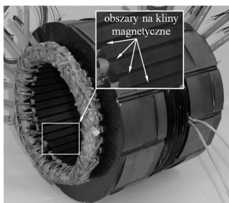
Rys. 2. Stojany i dodatkowa cewka maszyny ECPSM
