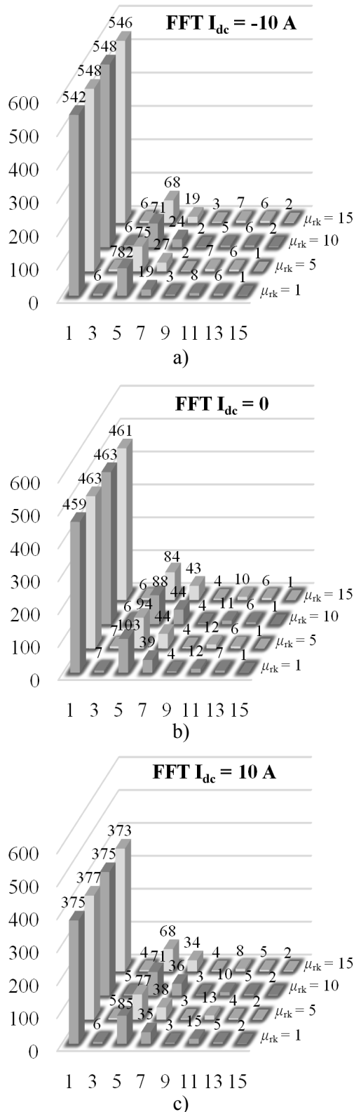
Rys. 11. Rozkład wyższych harmonicznych napięcia indukowanego
