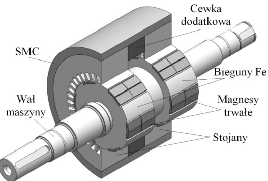
Rys. 1. Widok części aktywnych maszyny ECPSM
