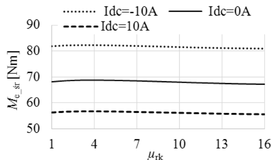
Rys. 7. Wartość średnia momentu elektromagnetycznego w funkcji \mu_{rk}
