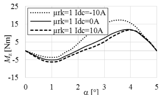
Rys. 3. Przebieg momentu zaczepowego przy \mu_{rk} = 1
