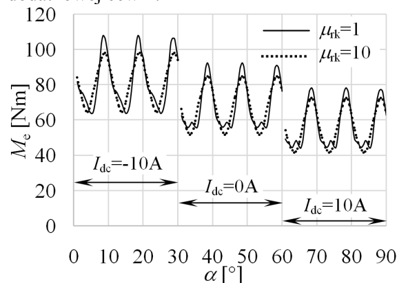
Rys. 6. Moment elektromagnetyczny bez klinów magnetycznych ( \mu_{rk} = 1 ) oraz z klinem ( \mu_{rk} = 10 ) dla trzech stanów wzbudzenia prądem dodatkowej cewki
