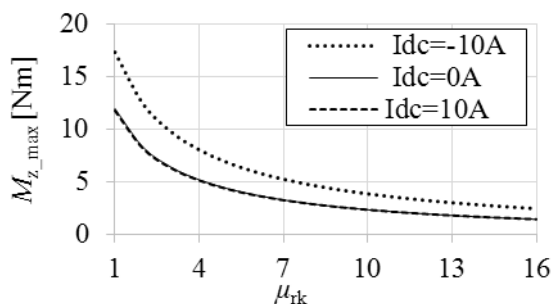
Rys. 5. Zależność wartości maksymalnej momentu zaczepowego w funkcji przenikalności klinów dla trzech stanów wzbudzenia prądem dodatkowej cewki
