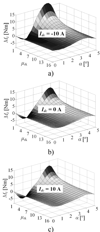
Rys. 4. Moment zaczepowy w funkcji przenikalności klinów i kąta położenia wirnika dla 3 stanów wzbudzenia prądem dodatkowej cewki
