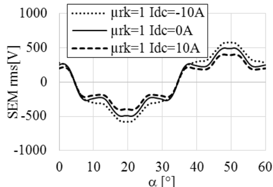
Rys. 9. Przykładowy przebieg napięcia indukowanego dla \mu_{rk}=1 przy prędkości wirnika n=3000 obr/min dla trzech stanów wzbudzenia prądem dodatkowej cewki
