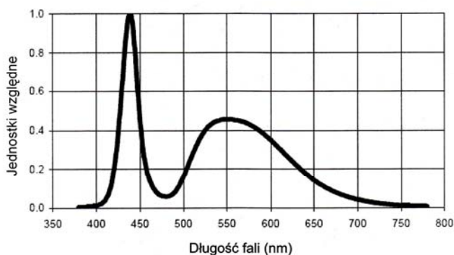
Rys. 1. Typowe widmo promieniowania diody LED o wysokiej temperaturze barwowej
