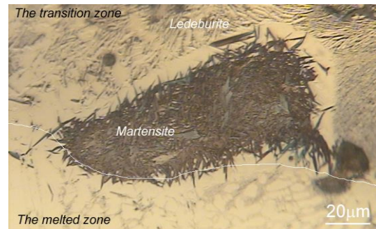
Fig. 4. The microstructure of the transition zone in the surface layer of malleable iron after laser heat treatment. Etched with nitride acid solution Rys. 4. Mikrostruktura strefy przejściowej w warstwie wierzchniej żeliwa ciągliwego po laserowej obróbce cieplnej. Trawione nitałem
