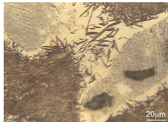
Fig. 4. The microstructure of the transition zone in the surface layer of malleable iron after laser heat treatment. Etched with nitride acid solution Rys. 4. Mikrostruktura strefy przejściowej w warstwie wierzchniej żeliwa ciągliwego po laserowej obróbce cieplnej. Trawione nitałem
