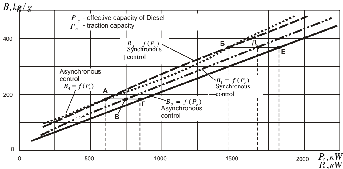
Fig. 2. Hourly consumption of fuel at the synchronous and asynchronous control by Diesel-generators Рис. 2. Часовой расход топлива при синхронном и асинхронном управлении дизель-генераторами
