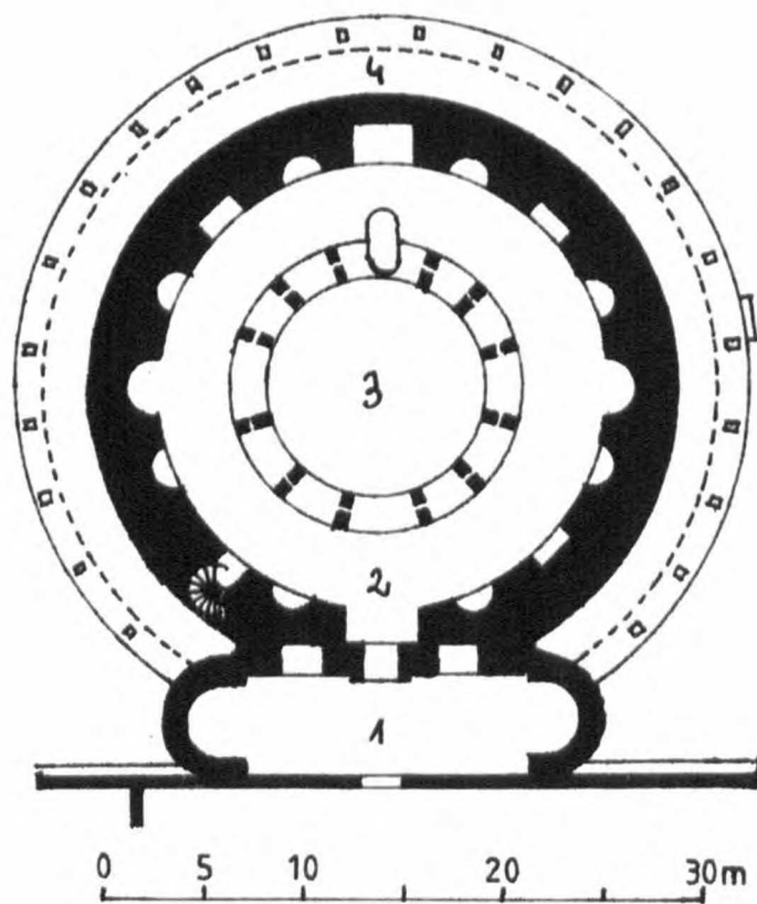
5. Rzym. Mauzoleum Konstantyny (ok. 330 r.) – plan: 1 – narteks (westybul); 2 – obejście; 3 – aulă z wieńcem kolumn; 4 – portyk kolumnowy
